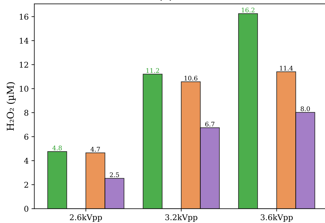
(d) \text{H}_2\text{O}_2
